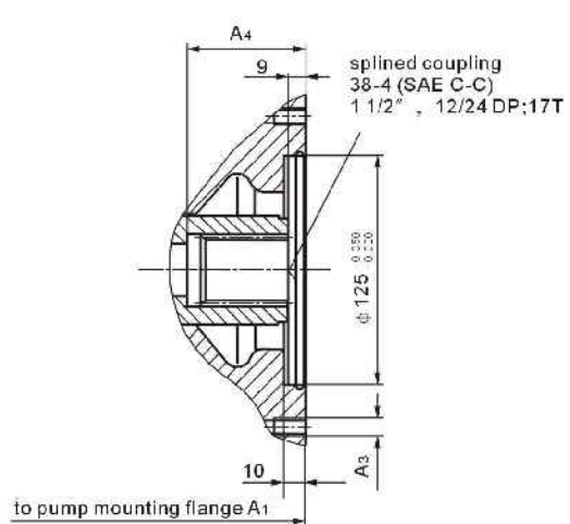
section A-B
