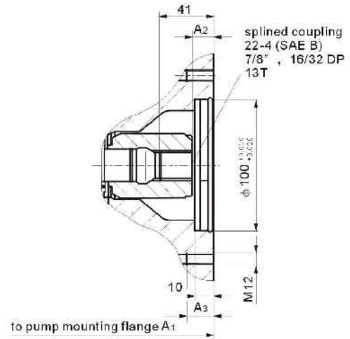
section A-B
