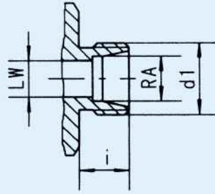
DIN 2353 LR
