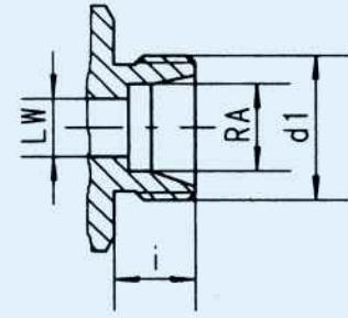
DIN 2353 SR
