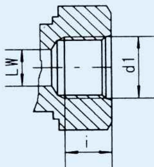
SAE J 514
