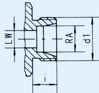
DIN 2353 SR
