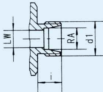
DIN 2353 LR
